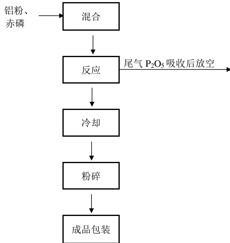
图 2.4.2 工艺流程简图
